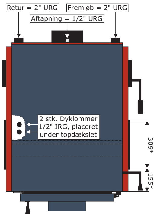
Set ovenfra
