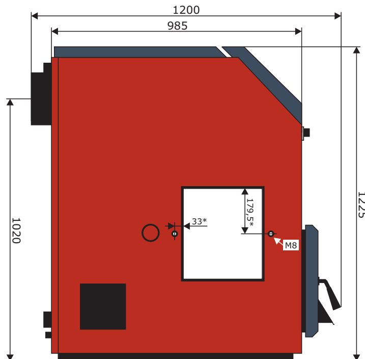
KA 4120 Alcon 3A-50 Dobbelt flange model - Set fra venstre side
