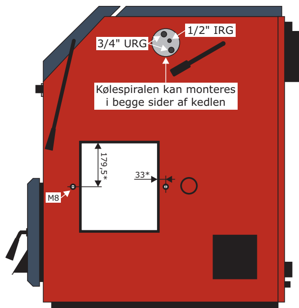
KA 4120 Alcon 3A-50 Dobbelt flange model - Set fra højre side
